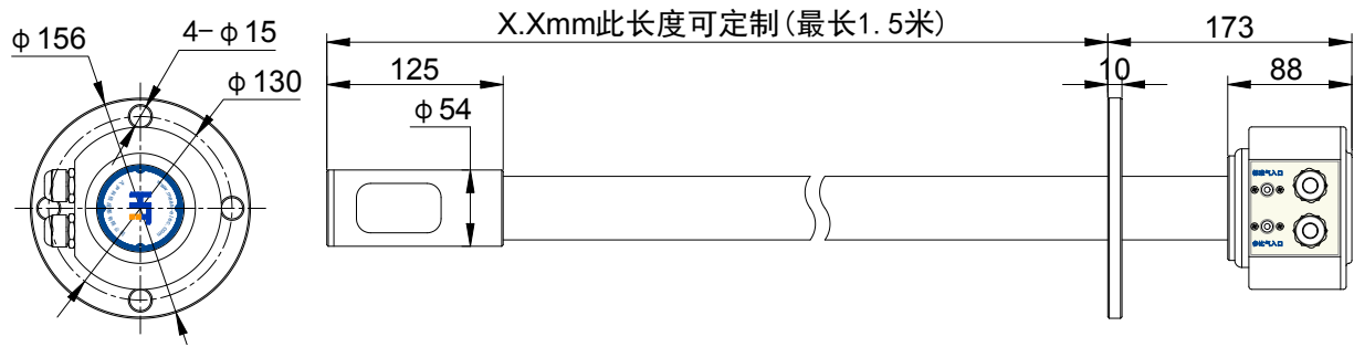
探头部分
