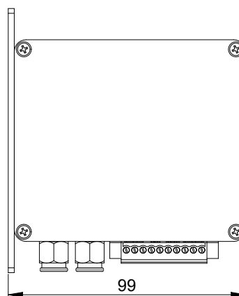
左视图
