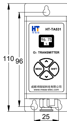
主视图
