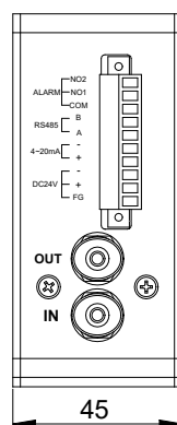
仰视图
