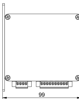
左视图
