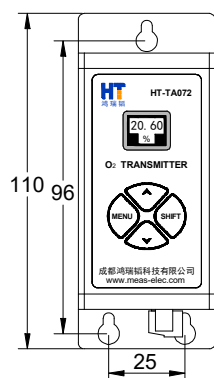
主视图
