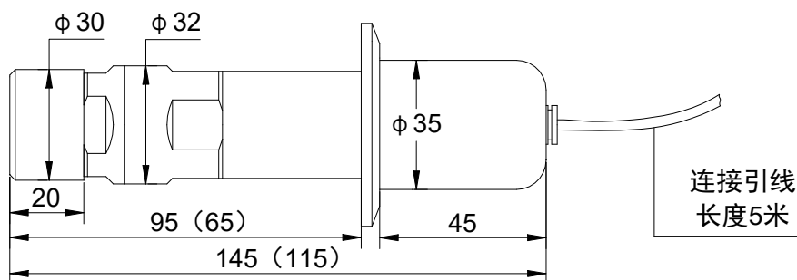
主视图
