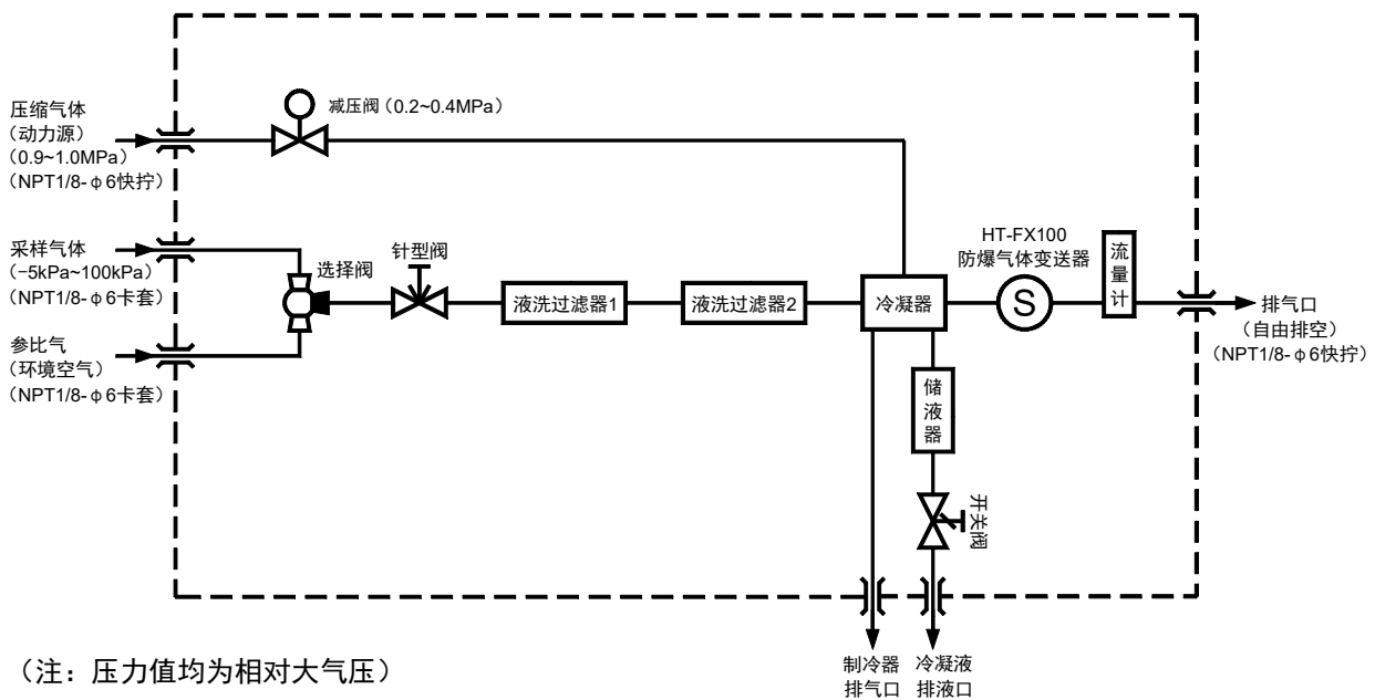
正压气路连接图
