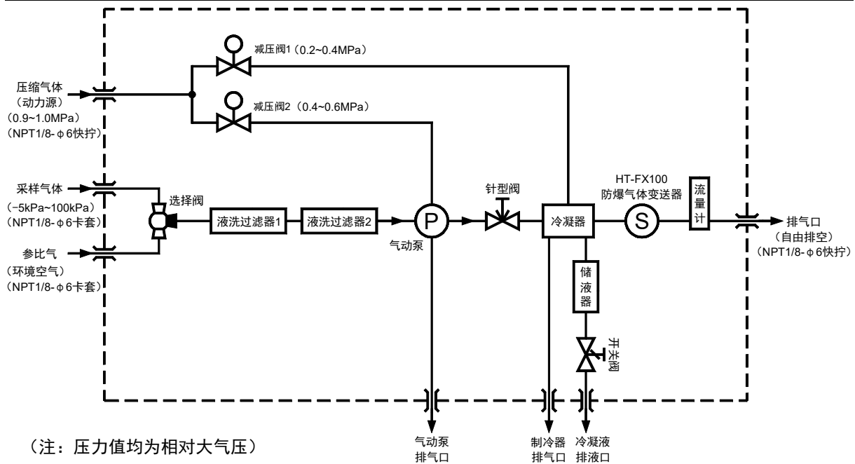
微正压、负压气路连接图
